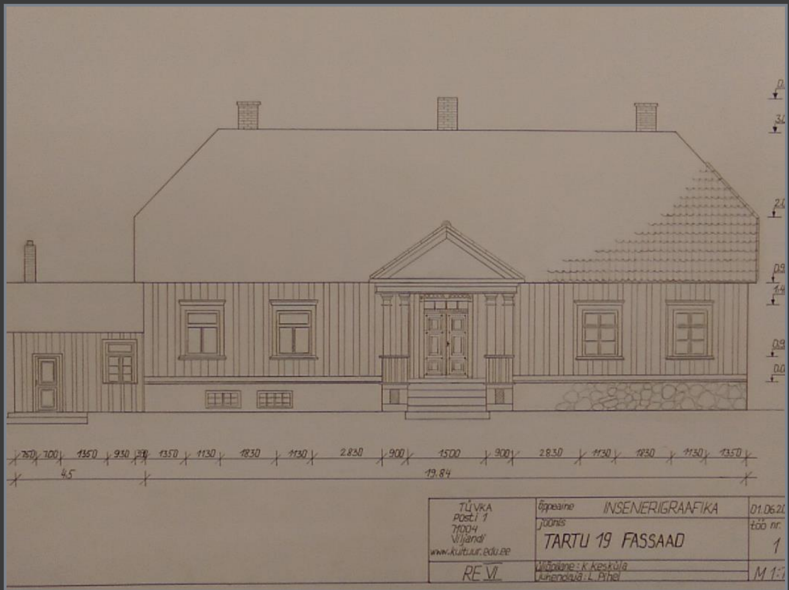
Viljandi, Tartu 19 fassaad. Insenerigraafika 2016. Juhendaja: Laur Pihel
