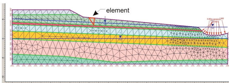
Joonis 2. Lõplike elementide meetodil põhinev mudel.
