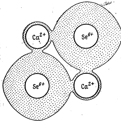
KERGELT KOVALENTNE IOONKRISTALL
