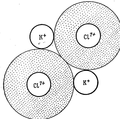
IOONKRISTALL (NaCl, KCl)
